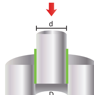
▲ Bonded Press Fit
